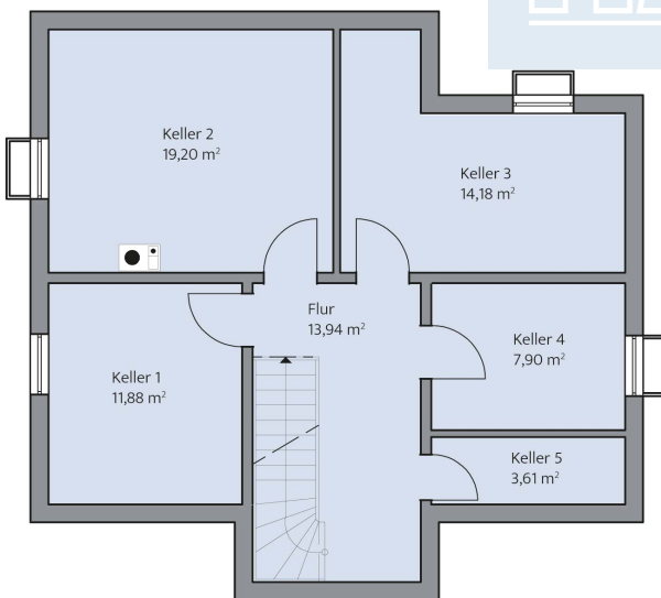
Haus Römer Grundriss
