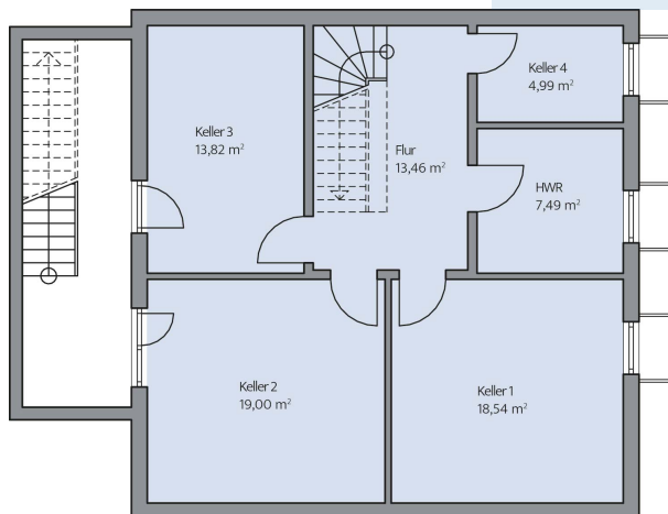
Haus Engelhardt Grundriss
